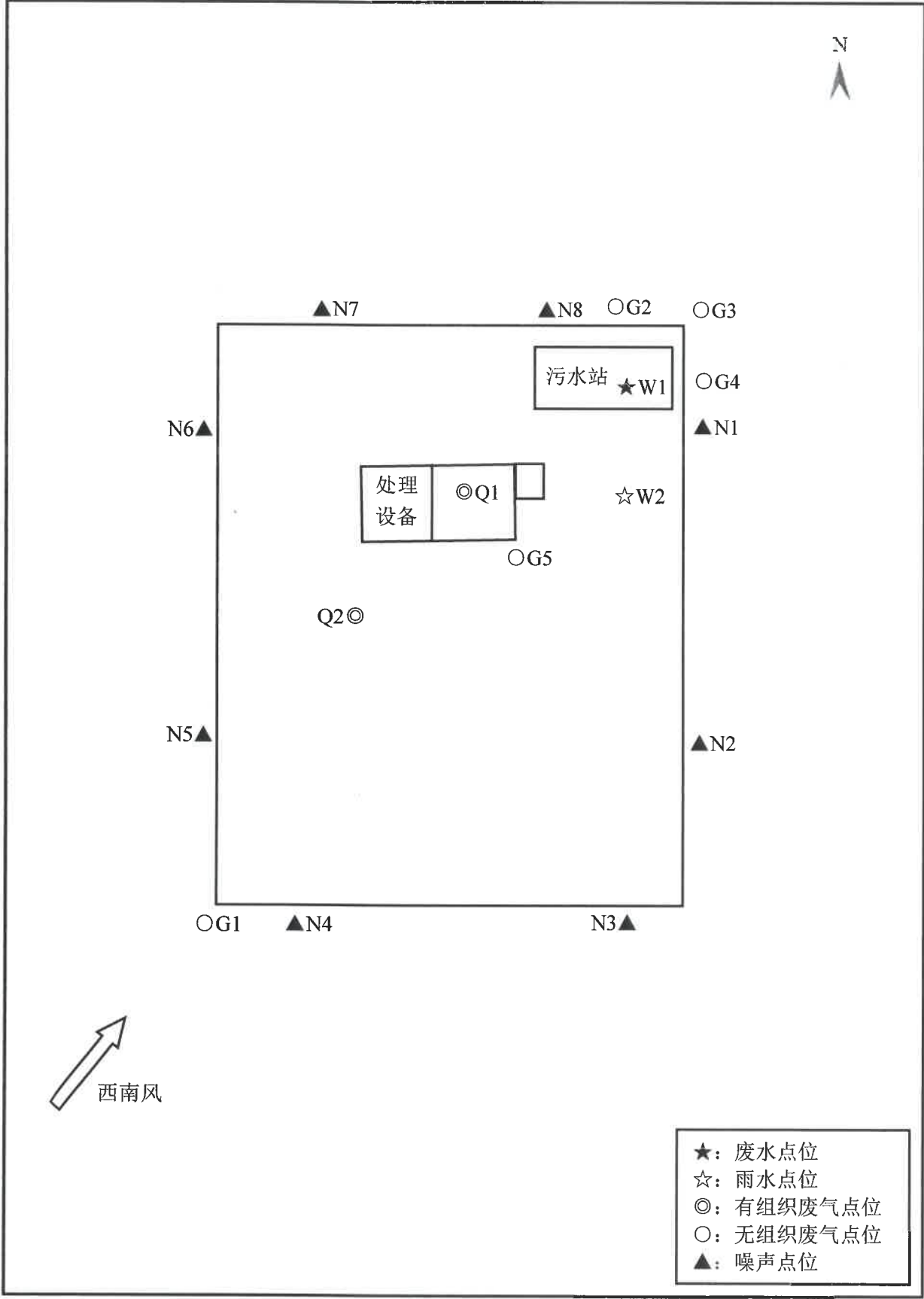
测点示意图
